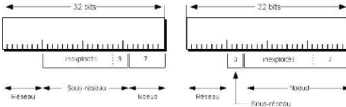
Figure 24.8 Réseaux – Sous-réseaux
