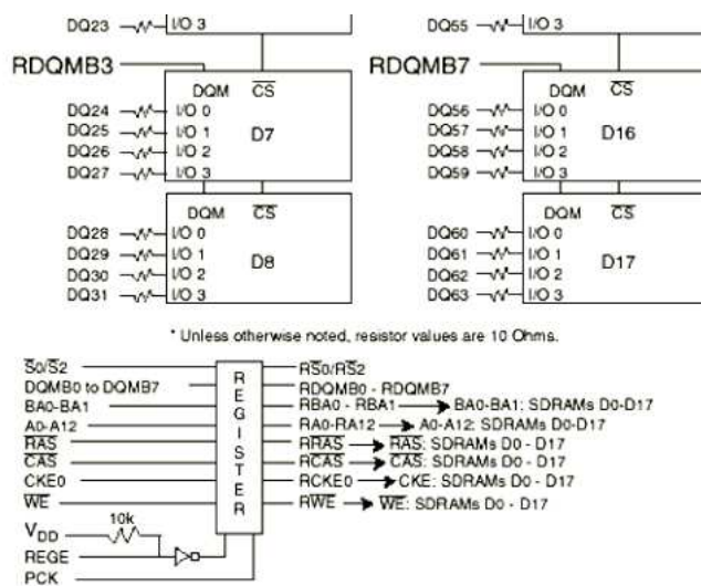
Figure 11.12 Extrait d'une implantation SDRAM 133 (doc. IBM)
