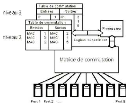
Figure 26.8 Le commutateur
