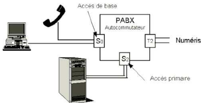
Figure 28.4 Accès Numéris
