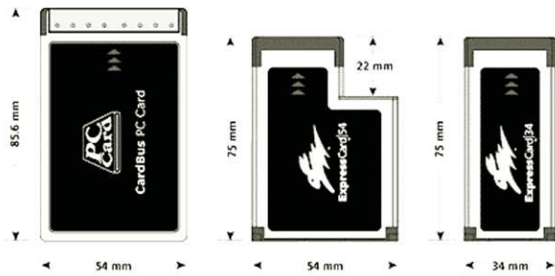
Figure 15.7 Les formats PCCard et Express Card
