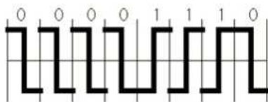
Figure 12.5 Mode PE
