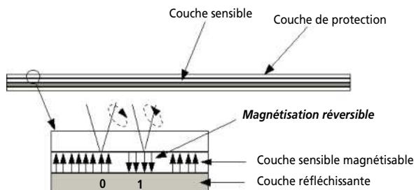
Figure 14.8 Principe du magnéto-optique
