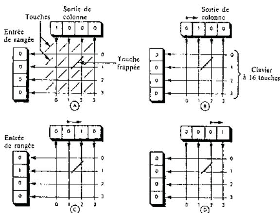
Figure 20.8 Identification de la touche par balayage des colonnes
