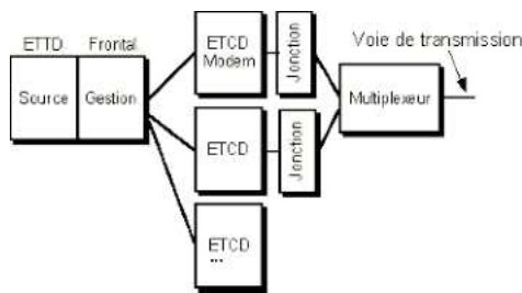
Figure 22.7 ETTD et ETCD
