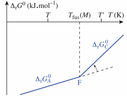
Doc. 5. Évolution de la courbe d'Ellingham \Delta_r G^0(T) lors de la fusion du corps simple : la pente du segment d'Ellingham augmente.
