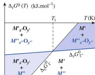
Doc. 18. Domaines de stabilité des oxydes M'_{x'} O_{y'} et M''_{x''} O_{y''} .
