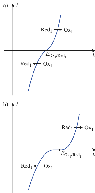
Doc. 5. Systèmes rapides et systèmes lents :
