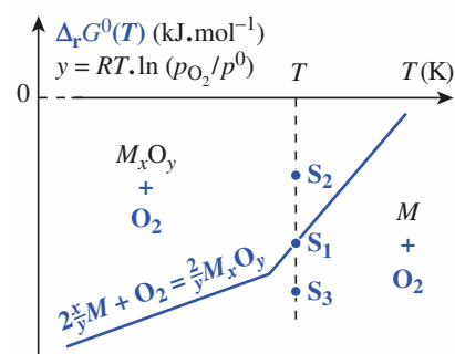
Doc. 9. Domaines de stabilité du corps simple M et de l'oxyde M_xO_y . En ordonnées sont portées les grandeurs \Delta_r G^0(T) et RT \cdot \ln(p_{O_2}/p^0) dont l'homogénéité est établie à la relation (6.8) (cf. aussi § 3.1.).
