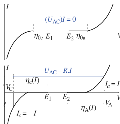
Doc. 18. Courbes intensité-potentiel pour les couples \text{Ox}_1/\text{Red}_1 et \text{Ox}_2/\text{Red}_2 .
