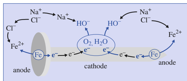
Doc. 36. Réactions électrochimiques ( \rightarrow ) et circulation des porteurs de charge ( \longrightarrow ) au cours de la corrosion du clou.
