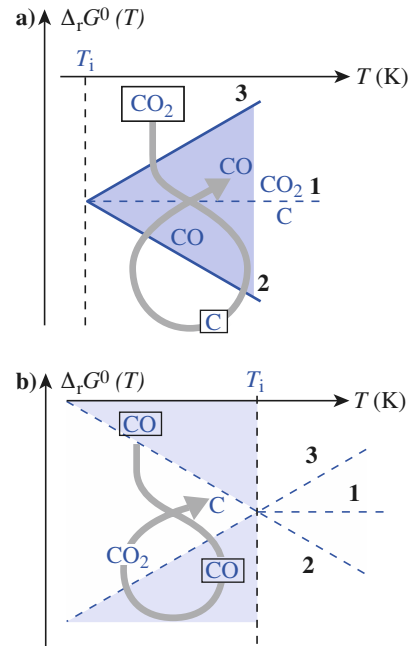
Doc. 22. Diagramme d'Ellingham du carbone et de ses oxydes, avec indication des domaines de stabilité de CO : a) pour T > T_i : médiamutation de C et \text{CO}_2 ; b) pour T < T_i : dismutation de CO.
