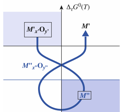
Doc. 19. Réduction spontanée de M'_{x'} O_{y'} par M'' .
