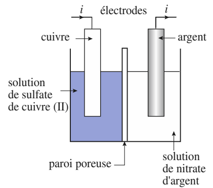
Doc. 4. Convention de représentation d'une cellule galvanique.
