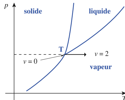
Doc. 1. Au point triple T ( v = 0 ), les trois phases solide, liquide et vapeur coexistent. Une élévation isobare de température provoque la disparition des phases solide et liquide : il y a rupture d'équilibre.
