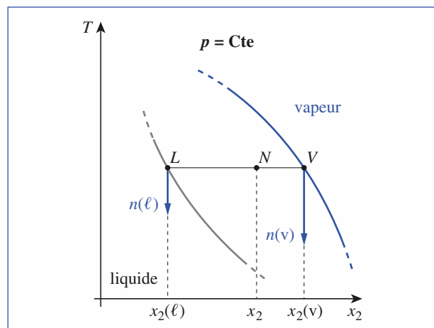
Doc. 14. Théorème des moments chimiques pour un système décrit à l'aide des fractions molaires. Les modules des vecteurs tracés sont proportionnels aux quantités de vapeur et de liquide :
