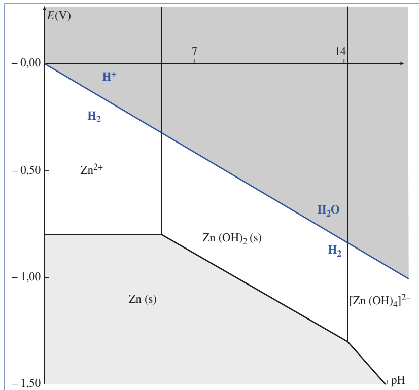
◀ Doc. 24. Diagramme E-pH du zinc à 25 °C pour C_{\text{tra}} = 1,0 \text{ mol} \cdot \text{L}^{-1} ; superposition du diagramme de l'eau.
