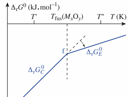
Doc. 6. Évolution de la courbe d'Ellingham \Delta_r G^0(T) lors de la fusion de l'oxyde : la pente du segment d'Ellingham diminue.
