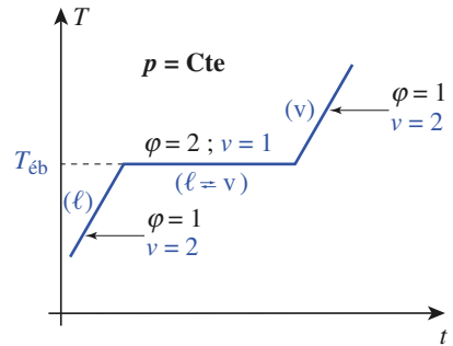
Doc. 2. Chauffage isobare d'un corps pur. Tant que le liquide et la vapeur coexistent, il y a équilibre entre les phases ( \nu = 1 ) et la température reste constante.
