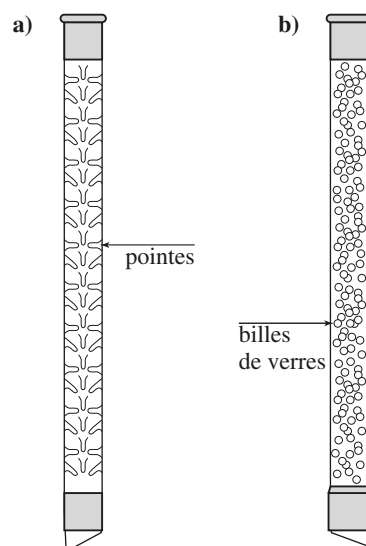
a) à pointes (colonne de Vigreux) ; b) à garnissage de verre (billes, tortillons...).
