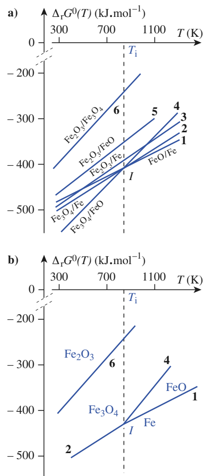
Doc. 25. Diagramme d'Ellingham du fer et de ses oxydes : a) courbes d'oxydation ; b) domaines de stabilité.
